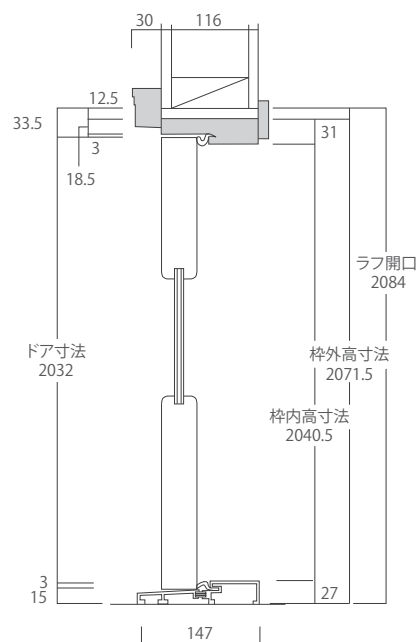
縦断面図
