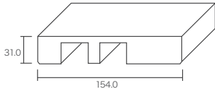
2本引き込み戸用 上部枠
