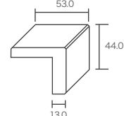
L型ケーシング 40
