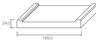
3本引き込み戸用 縦枠
