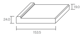
3本引き込み戸用 戸当
